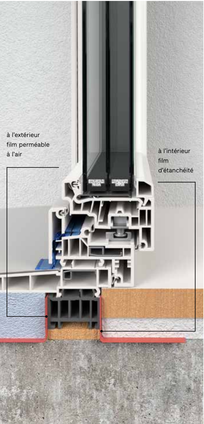
Pose en deux étapes avec précadre
