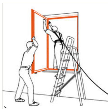
c Le nouveau dormant peut maintenant être vissé sur le précadre, et le nouvel ouvrant accroché.
