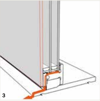
Socle tout en verre, évacuation d'eau invisible
