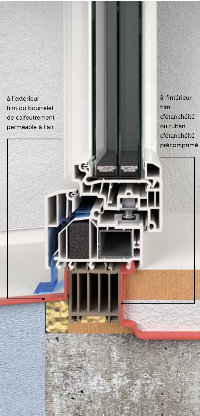
Pose en une étape directement sur la maçonnerie
