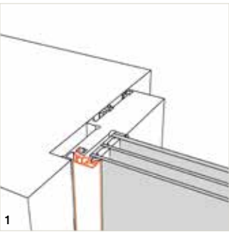
Cadre à peine visible
