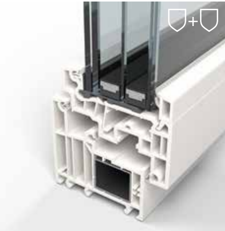
Vue en coupe d'une fenêtre avec triple vitrage isolant, verres extérieurs et intérieurs en exécution Multiprotect, configuration 44.2Sm-13-4F-13-66.2Sm
