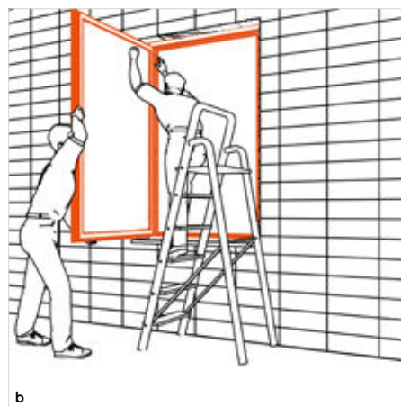
b Le cadre ouvrant est ensuite mis en place sur le dormant et l'installation est terminée.
